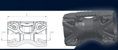
UNION DOUBLE À CLIPSER
