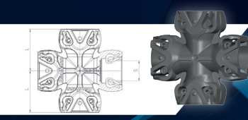
RACCORD EN CROIX 4 VOIES REGULAR
