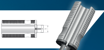
OUTILS DE DÉCONNEXION MÉTAL SYSTÈME
