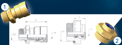
RACCORD UNION MÂLE FILETÉ
