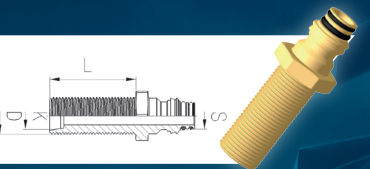
EMBASE FILETÉE CONIQUE LONG
