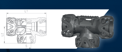
RACCORDS FORMET À CLIPSER
