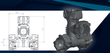
RACCORD BLOC 4 VOIES
