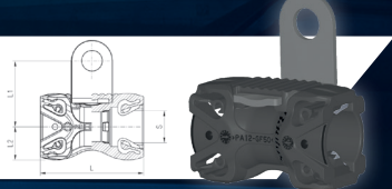
UNION DOUBLE À CLIPSER AVEC FIXATION
