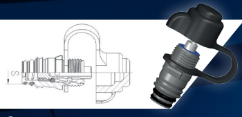
PRISE DE PRESSION À CLIPSER
